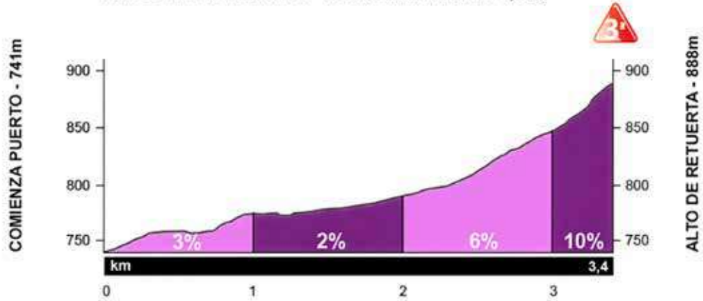
ALTO DE RETUERTA - Pendiente media: 4,3%
