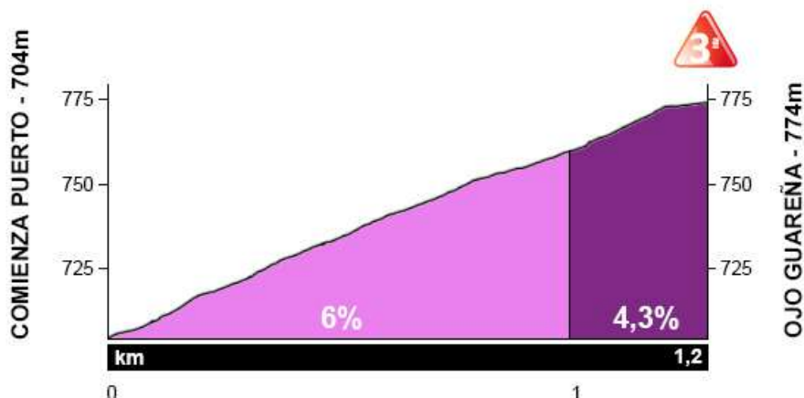
OJO GUAREÑA - Pendiente media: 5,8%
