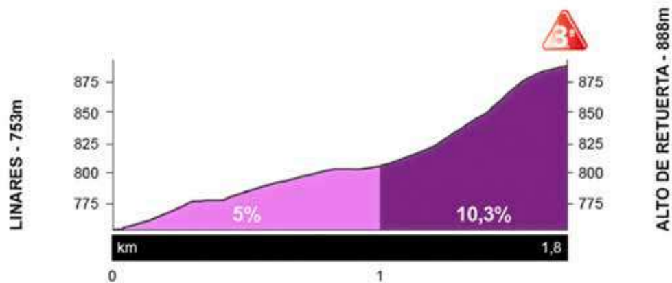
ALTO DE RETUERTA - Pendiente media: 7,7%
