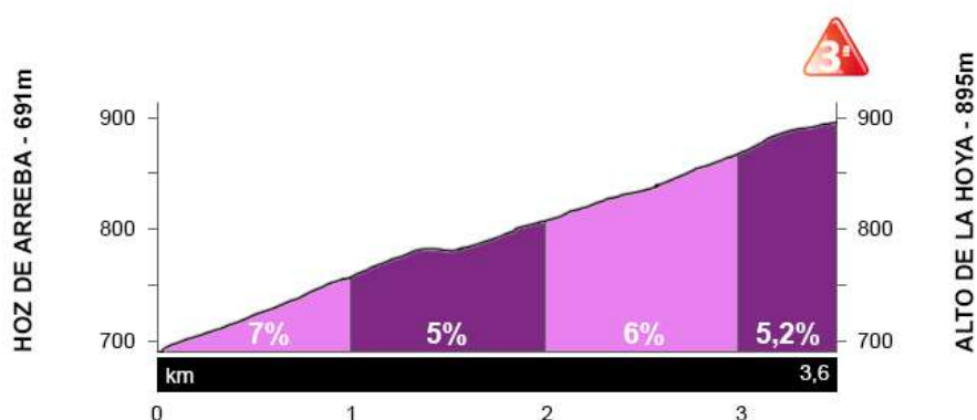
ALTO DE LA HOYA - Pendiente media: 5,7%
